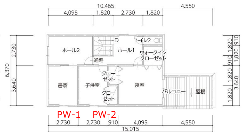
2階平面図
