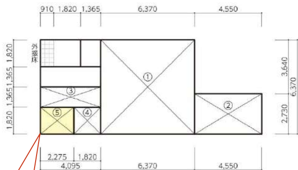
1階求積図
