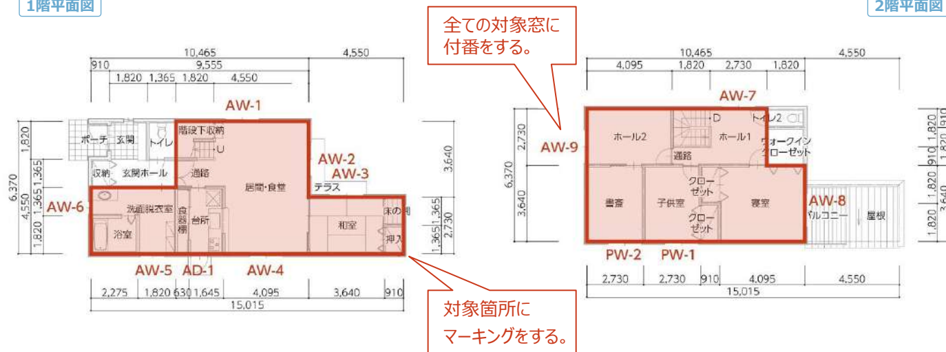
1階平面図
