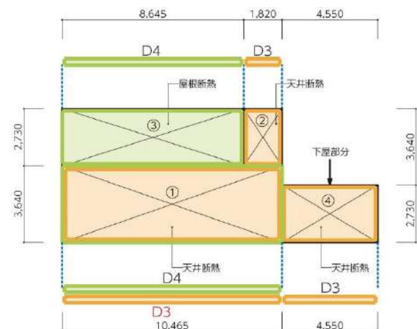
図2 天井求積図
