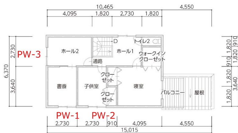
2階平面図
