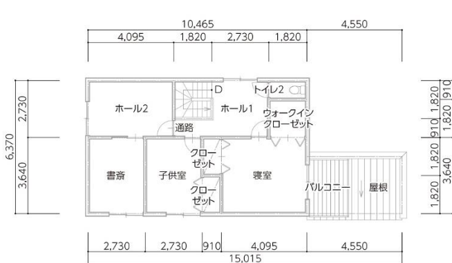
2階平面図
