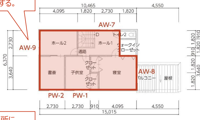
2階平面図
